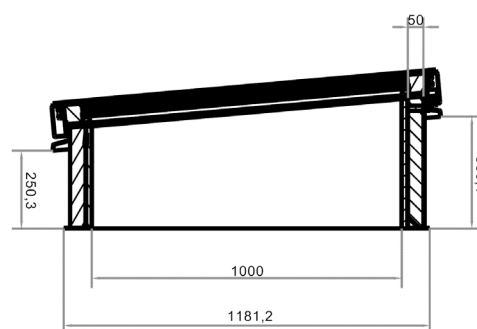
Dwarsdoorsnede
