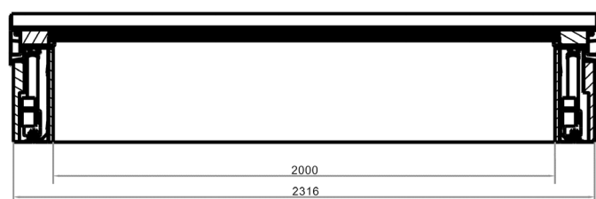
Langsdoorsnede
