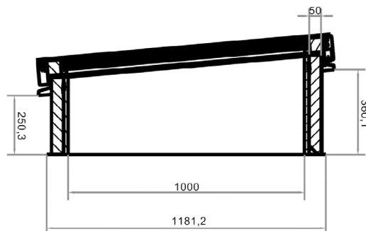
Dwarsdoorsnede
